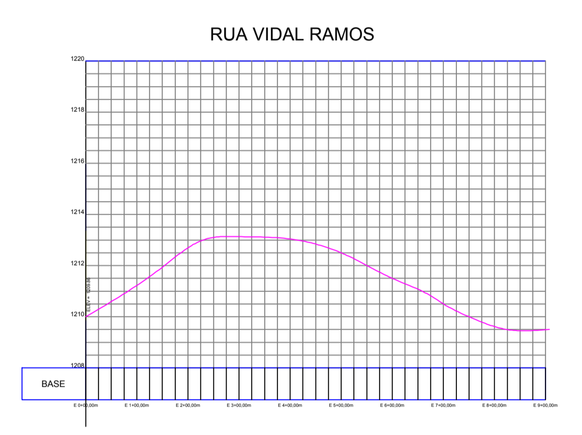
RUA VIDAL RAMOS PERFIL LONGITUDINAL Esc Vertical 1:75 Esc Horizontal 1:750
