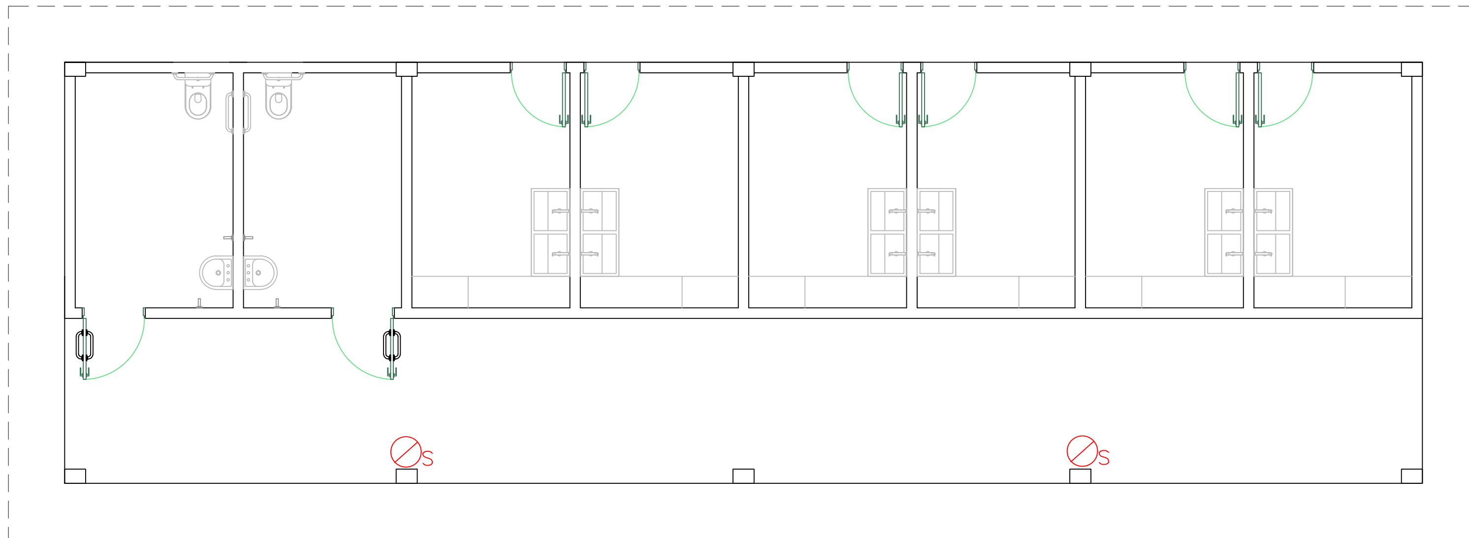
1 PLANTA BAIXA - ÁREA 116,10 M 2 ESCALA 1/75
