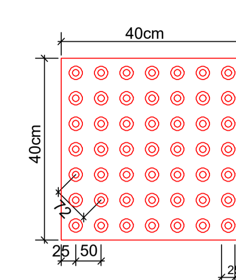
PISO TÁTIL ALERTA (40x40cm)
