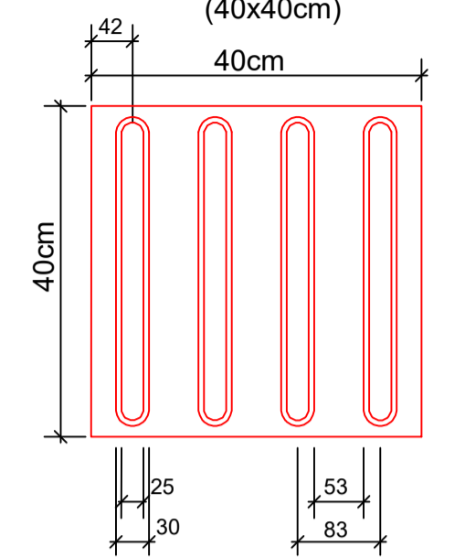
PISO TÁTIL DIRECIONAL (40x40cm)
