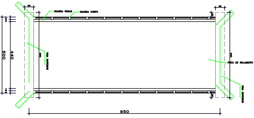
PLANTA BAIXA C/ DIMENSÕES ESC.:.....1:50 ÁREA=47,50m 2
