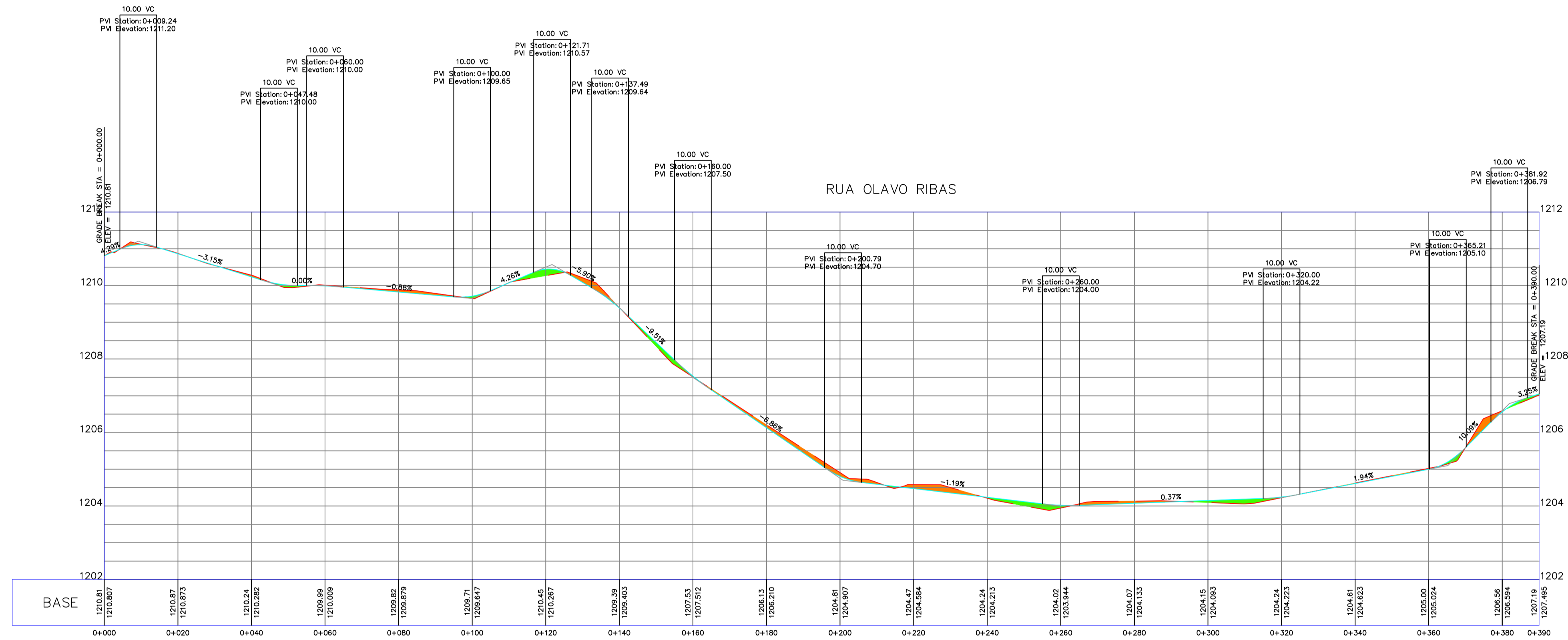
PERFIL LONGITUDINAL Escala Horiz. 1/750 Escala Vert. 1/75
