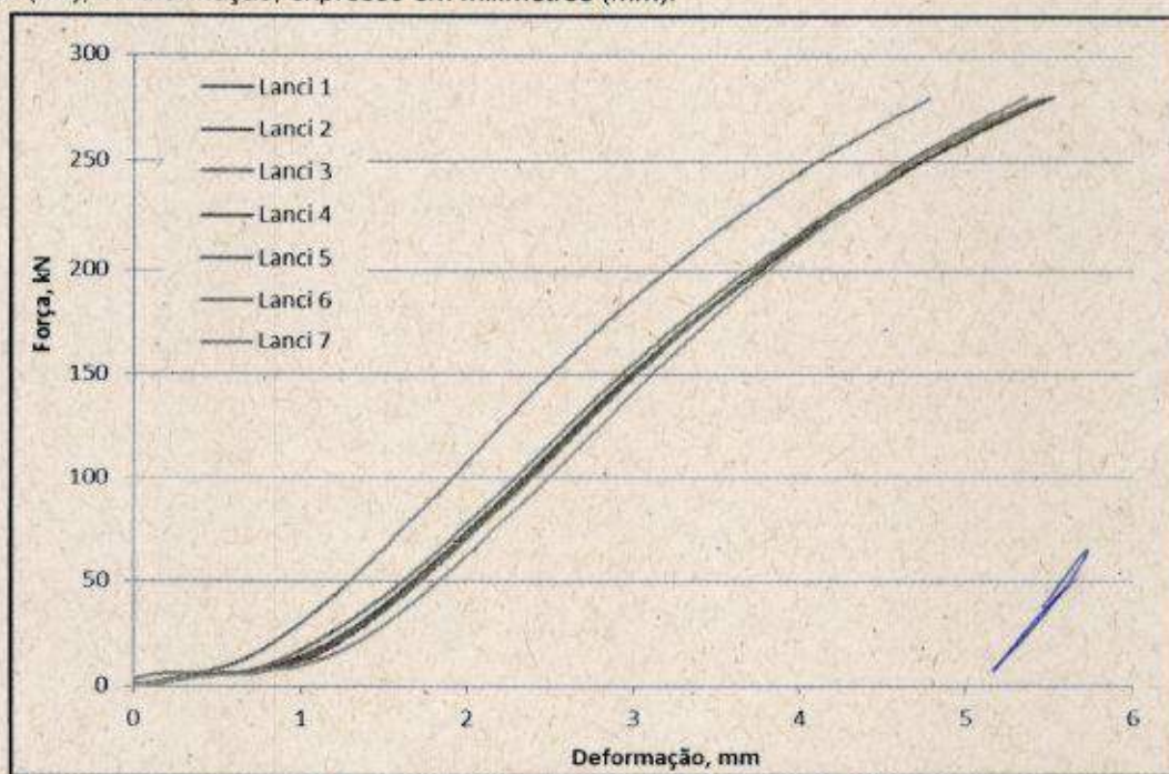
Figura 3 – Gráfico de Força x Deformação
