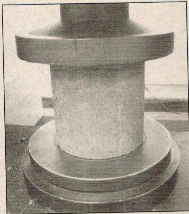
Figura 2 – Corpo de prova posicionada para ensaio
