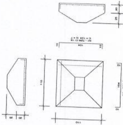
Sapata - Detalhe Armadura Escala 1/25
