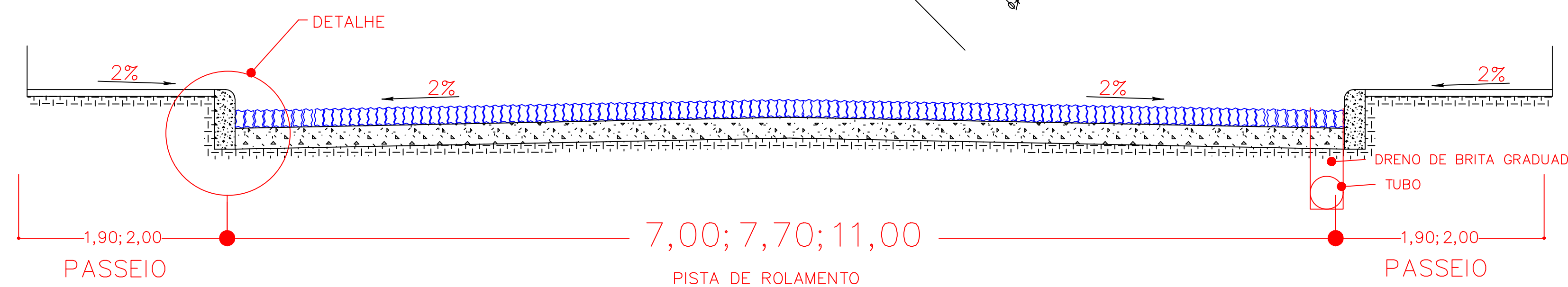
SEÇÃO TRANSVERSAL DO PAVIMENTO SEM ESC.
