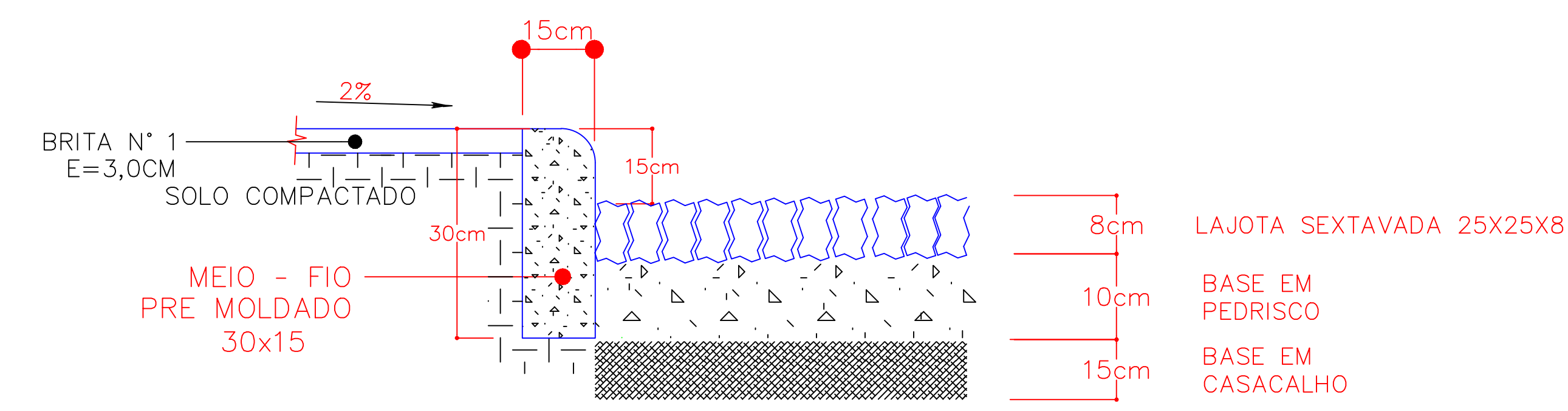
DETALHE ESC. 1/10
