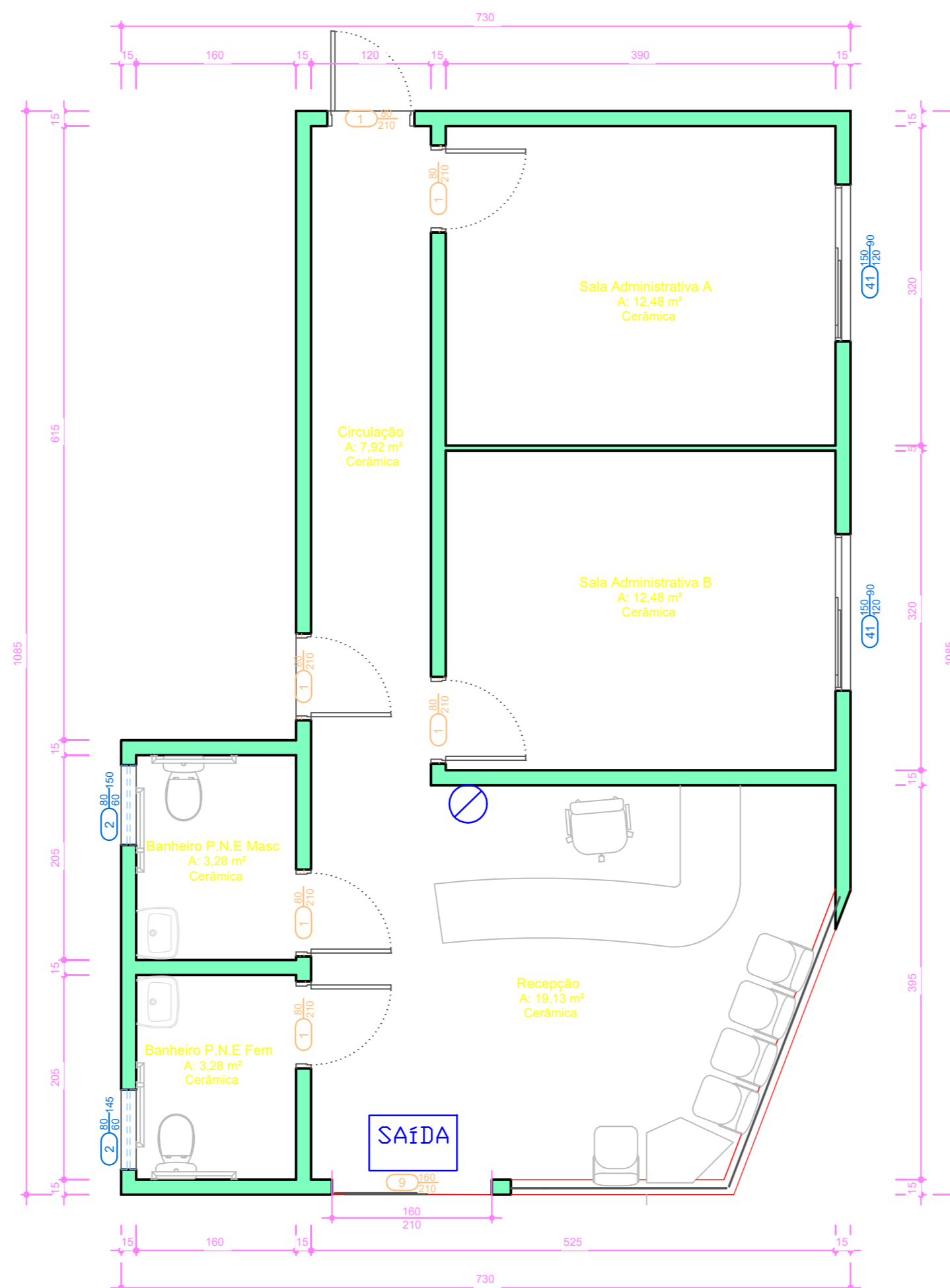
1 Planta Baixa - Bloco B Escala 1 : 50 Área: 66,40m 2
