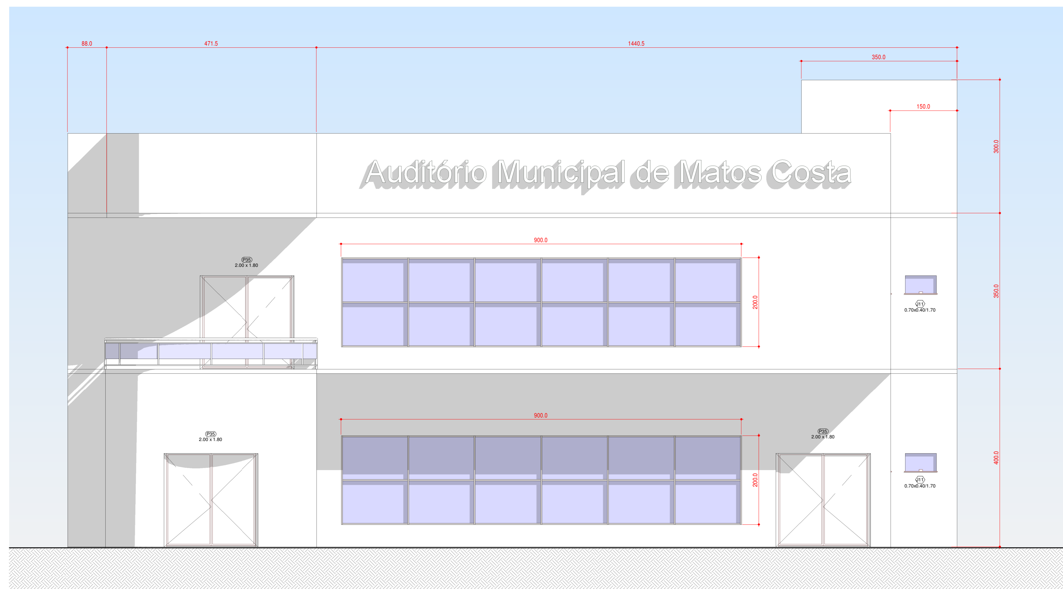
3 FACHADA DIREITA 1:50
