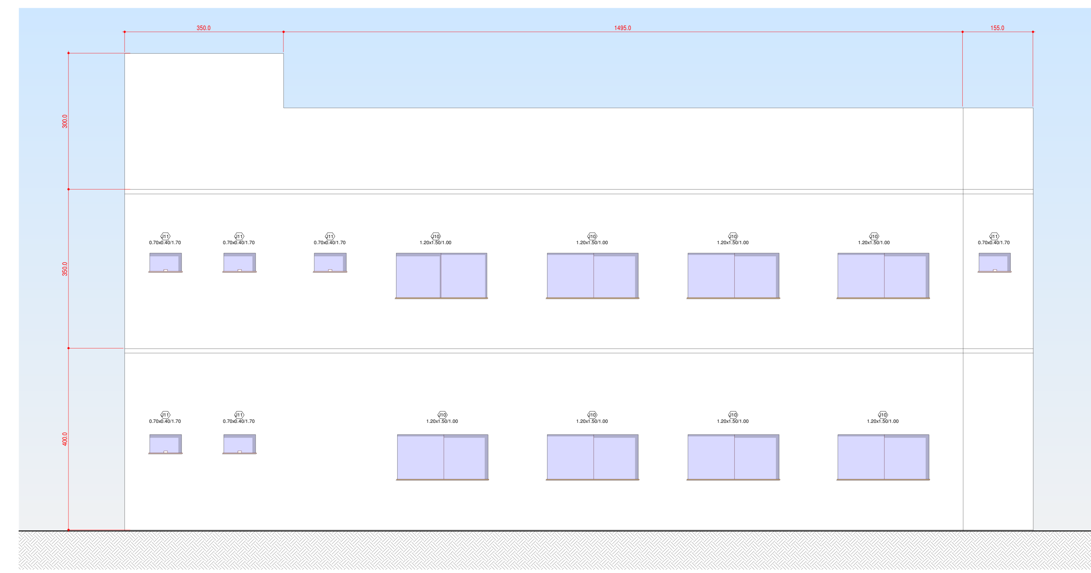
4 FACHADA ESQUERDA 1:50
