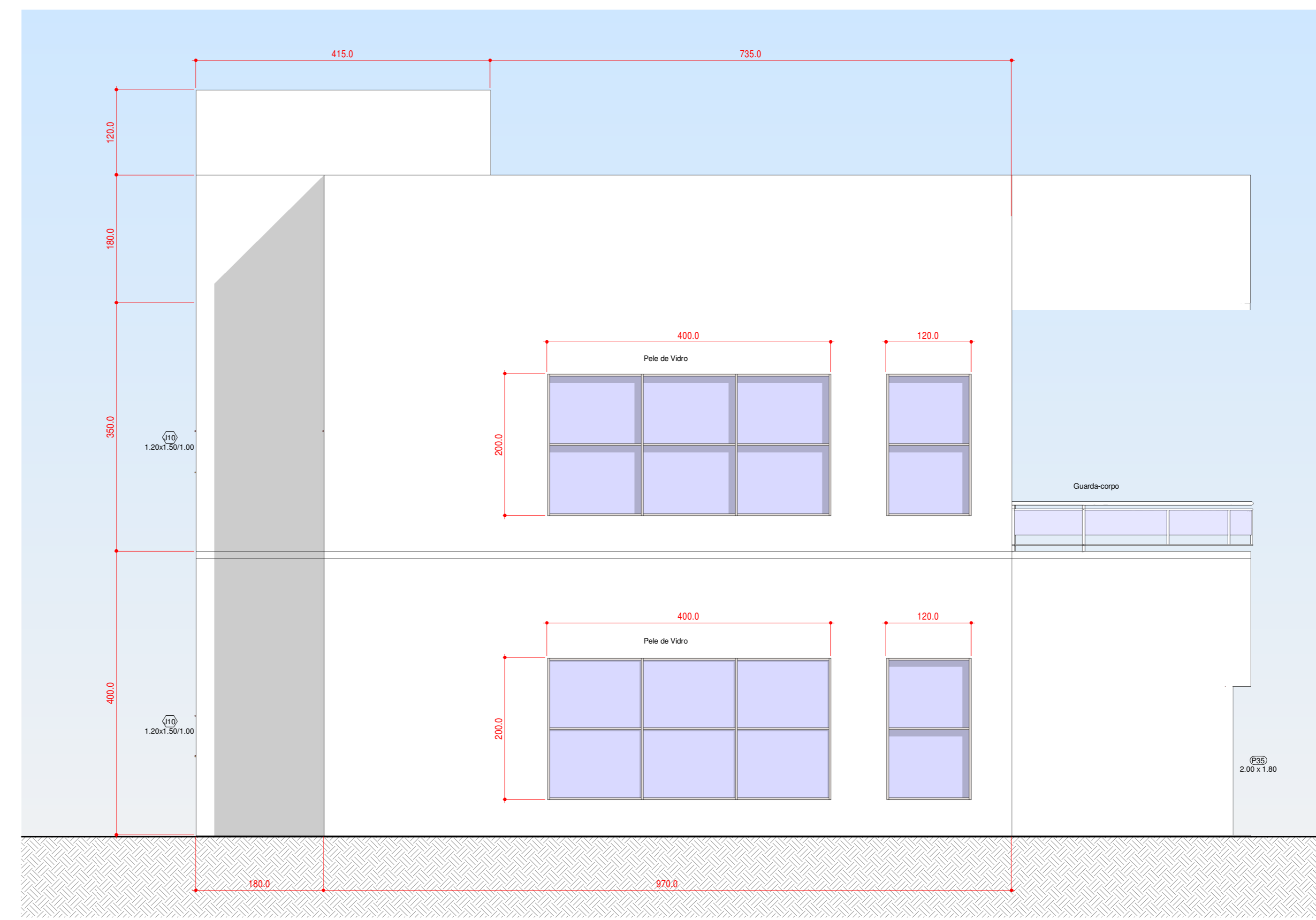
2 FACHADA FRONTAL 1:50
