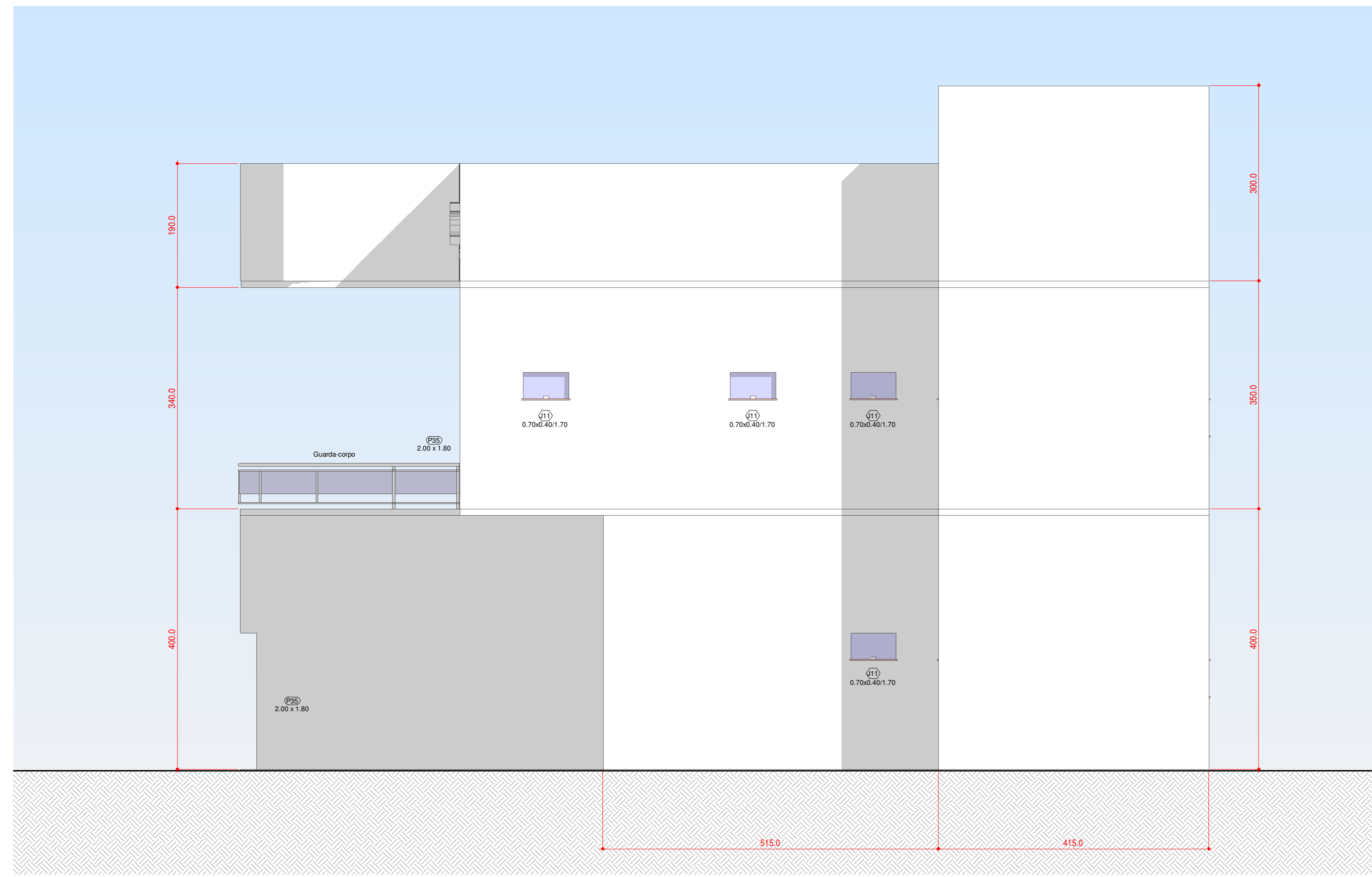
1 FACHADA POSTERIOR 1:50
