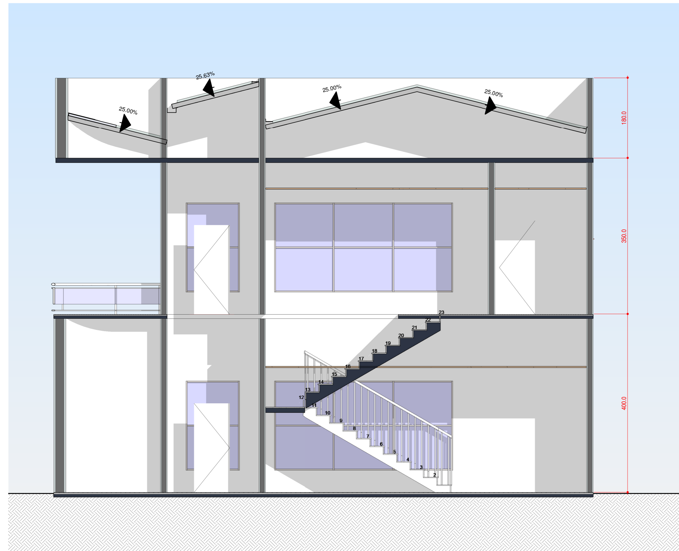
1 AA 1:50
