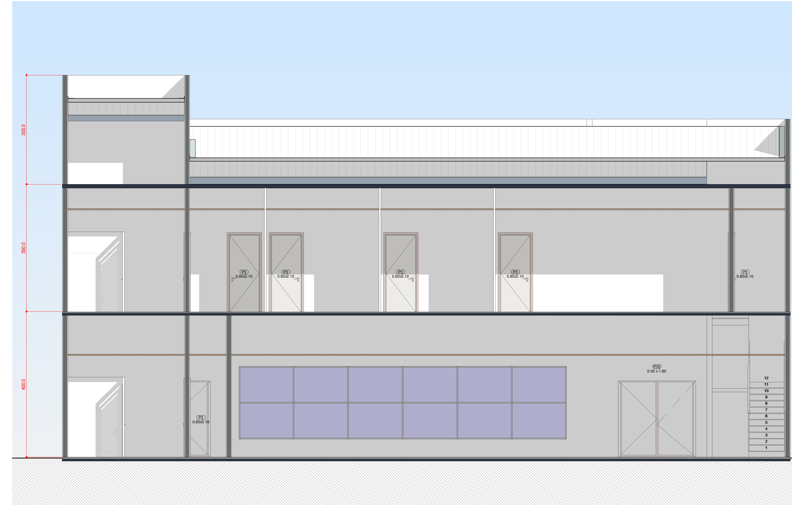
2 BB 1:50
