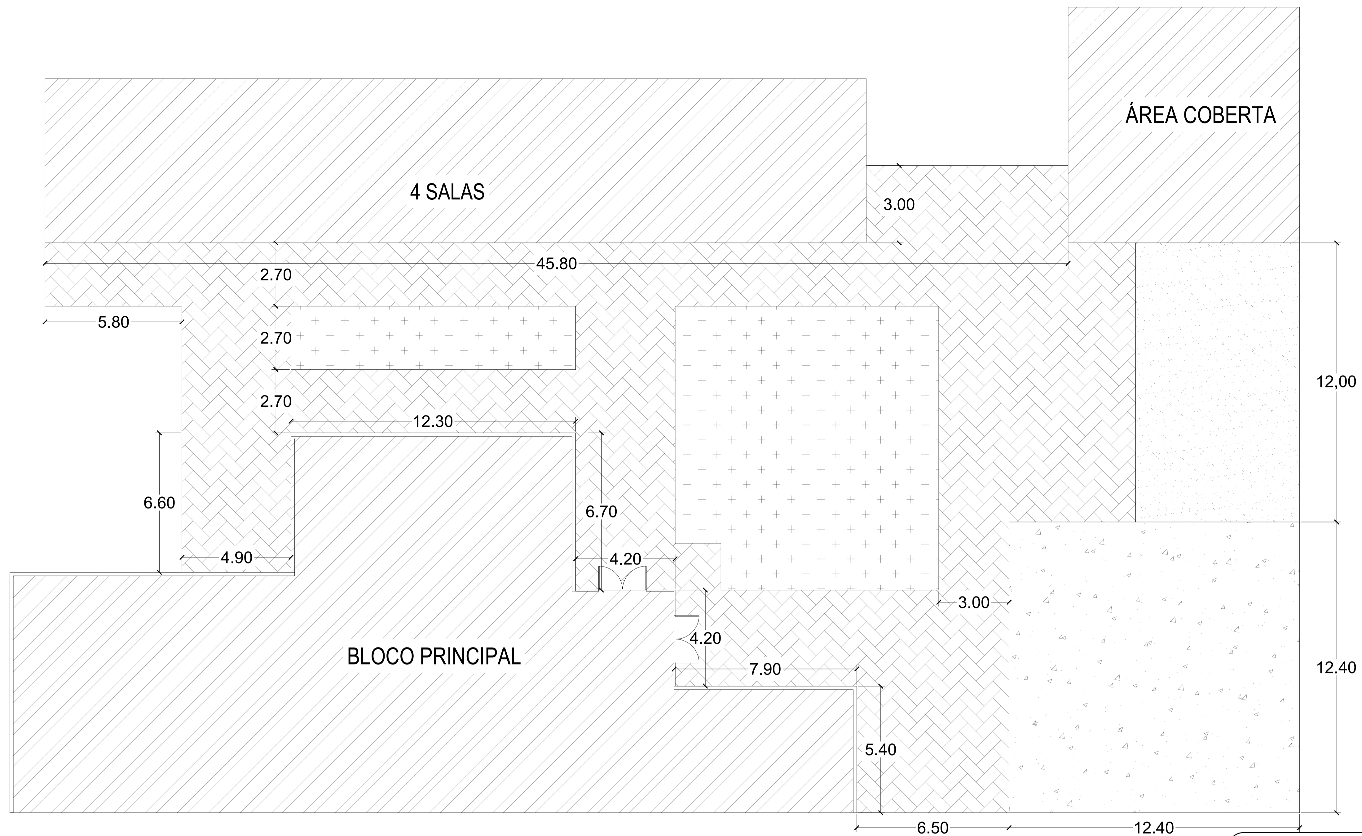
1 ÁREA DE IMPLANTAÇÃO ESCALA 1:100
