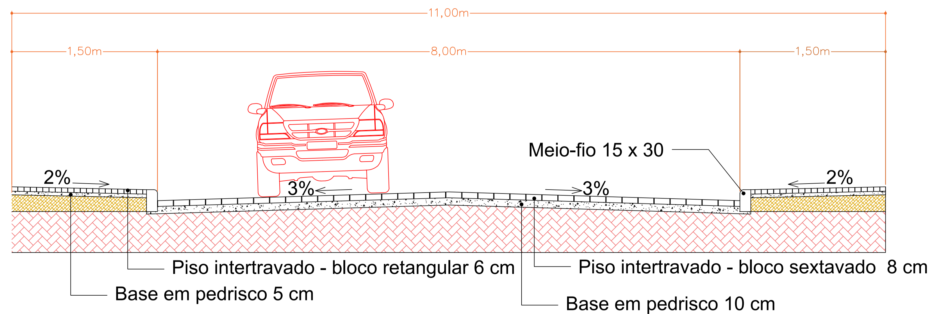
SEÇÃO TRANSVERSAL DO PAVIMENTO Sem Escala
