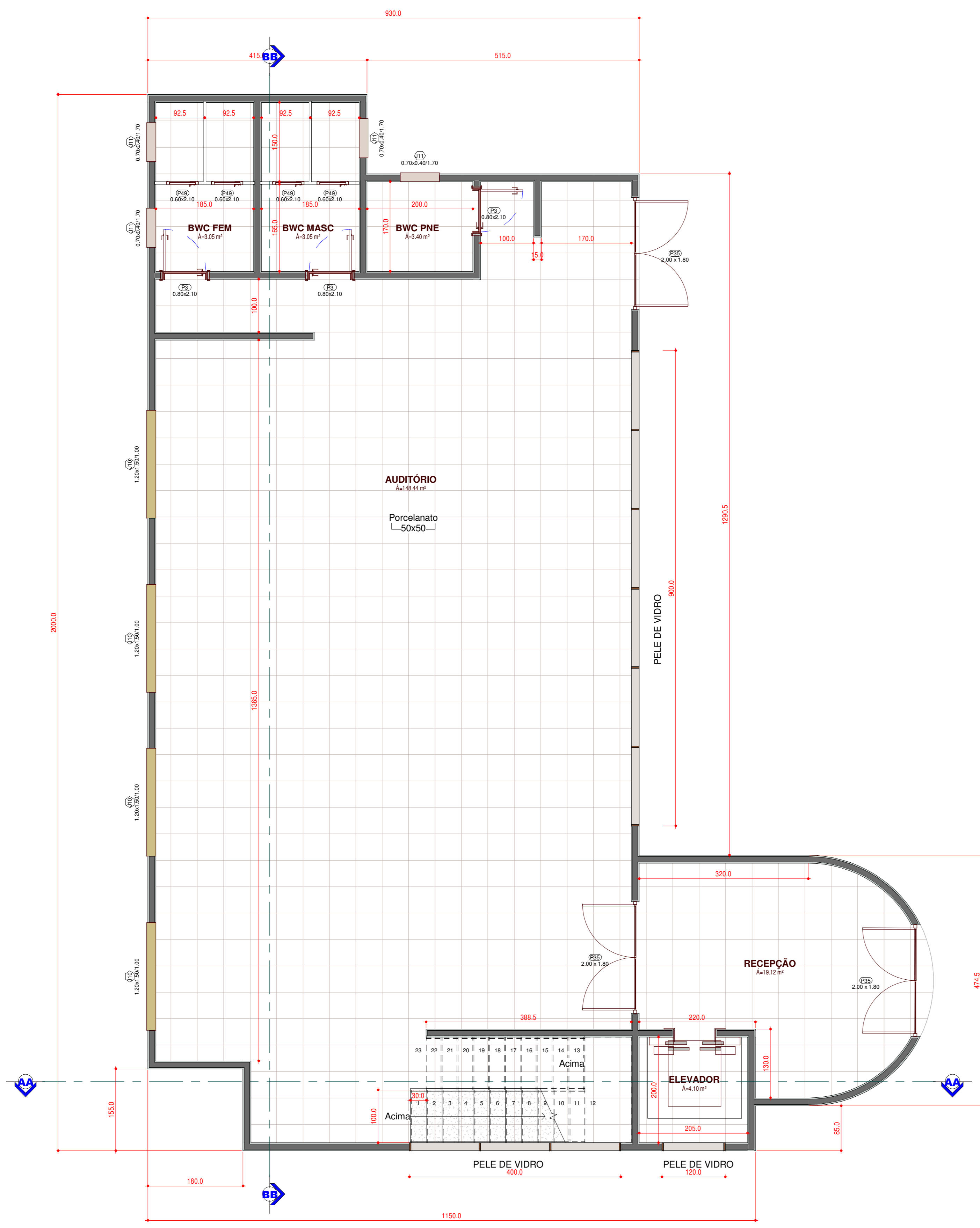
1 PLANTA FINAL - TÉRREO 1 : 50
